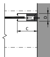
DETAIL UPEVNĚNÍ VODÍCÍCH LIŠT DO OTVORU
