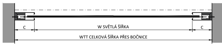
PŮDORYS - UPEVNĚNÍ DO OTVORU
