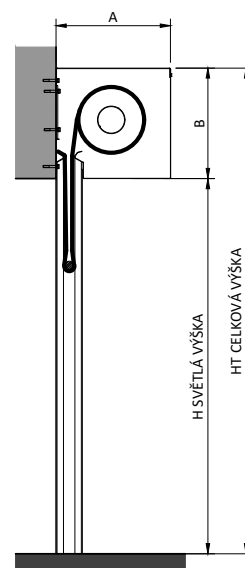
TYPICKÝ ŘEZ NA OTVOR
