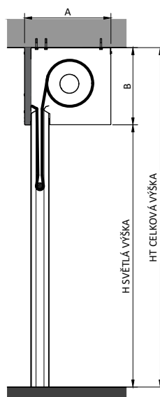
TYPICKÝ ŘEZ DO OTVORU
