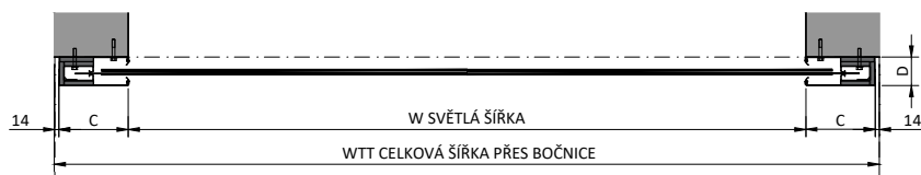
PŮDORYS - UPEVNĚNÍ NA OTVOR
